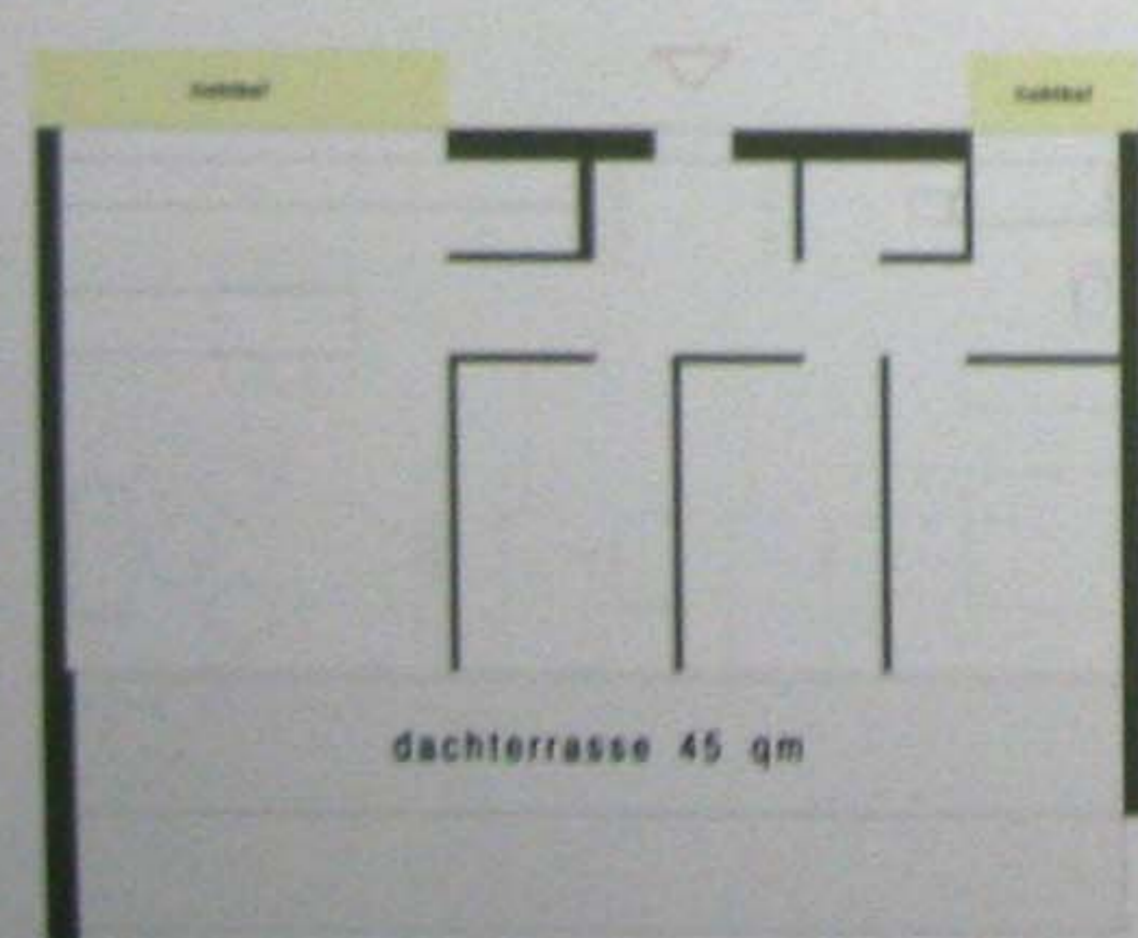
TYP E 4-ZIMMER 89 qm 1 : 100
