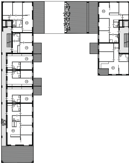
4. OG Wohnen "Bestand", Wohnen "Mitte" & Studentenheim M 1:200
