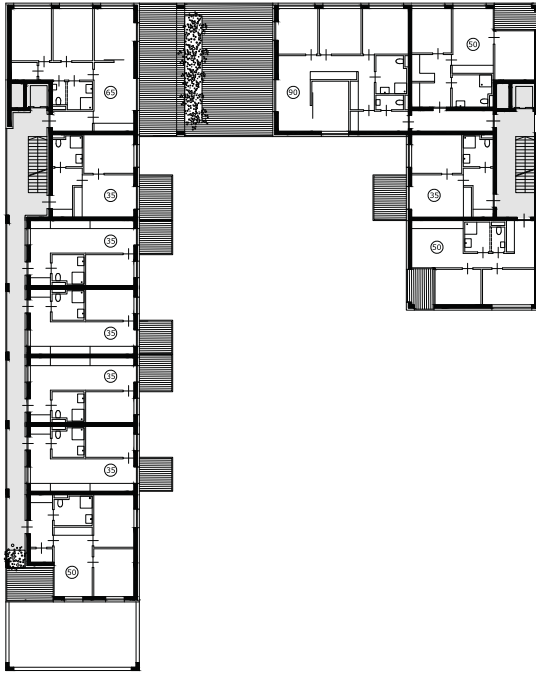
3. OG Wohnen "Bestand", Wohnen "Mitte" & Studentenheim M 1:200
