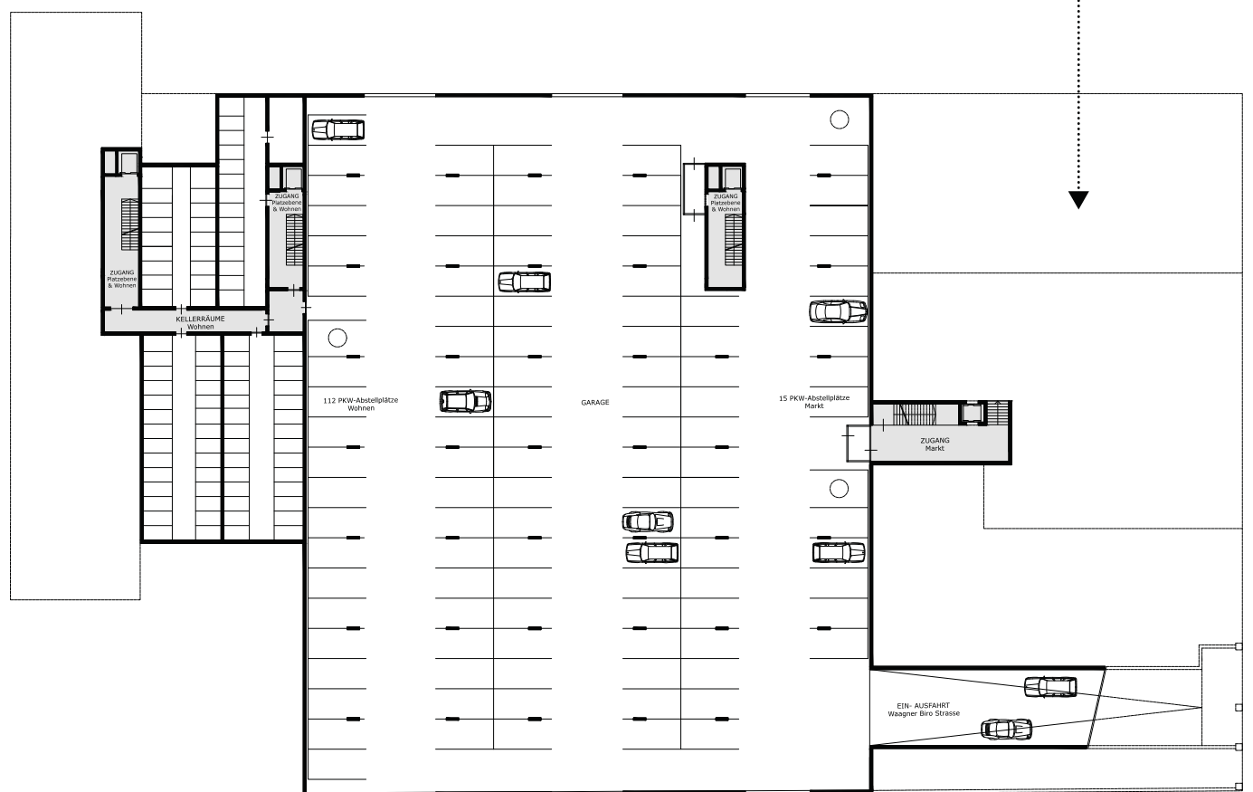
SOCKEL Garage & Kellerräume M 1:200
