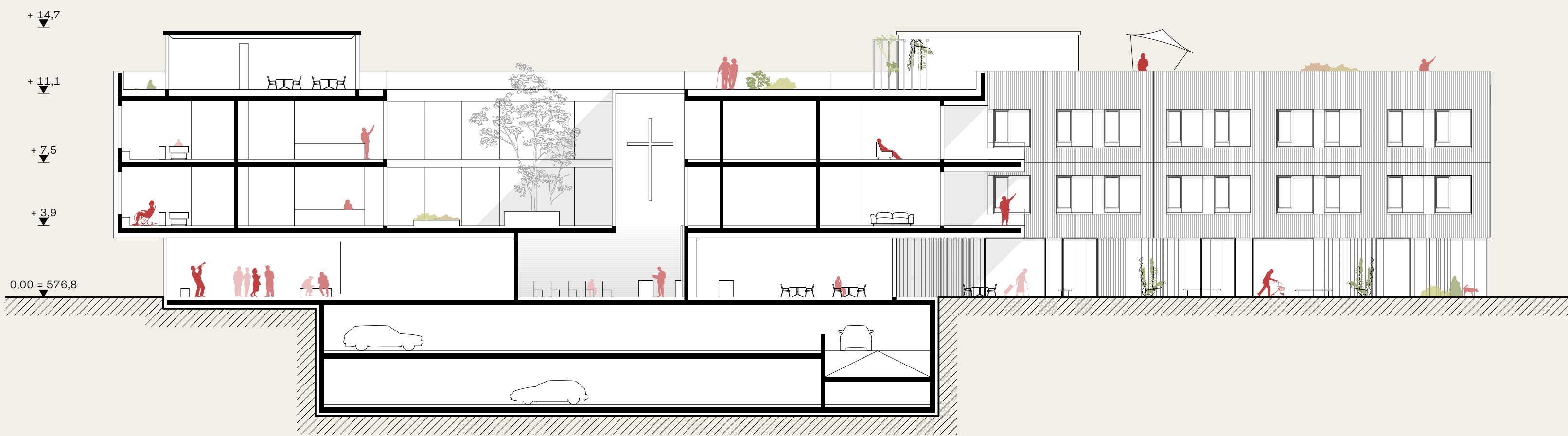
Schnitt | 1:200
