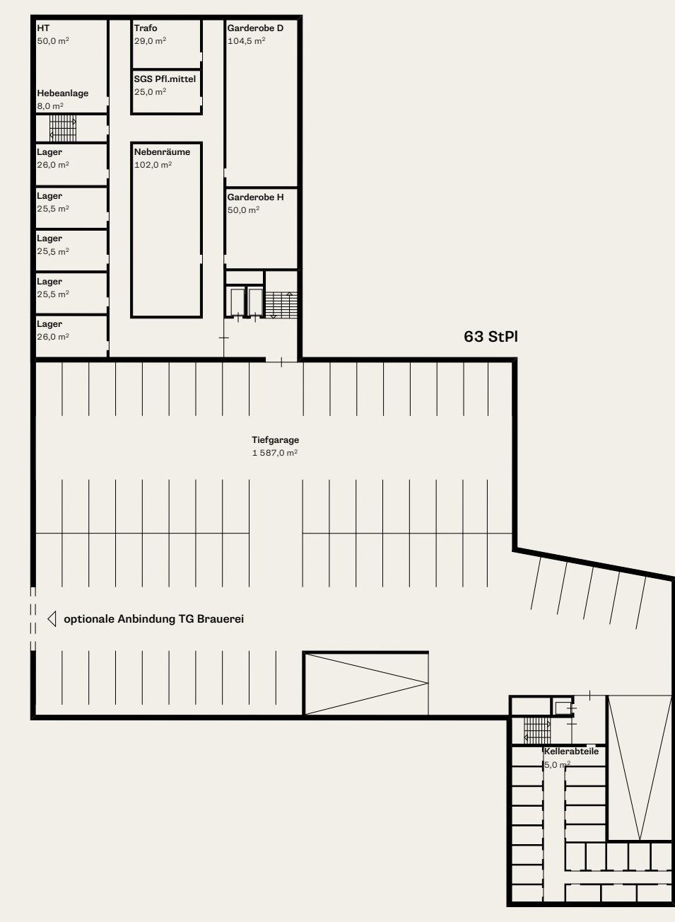
UG 1 | 1:500
