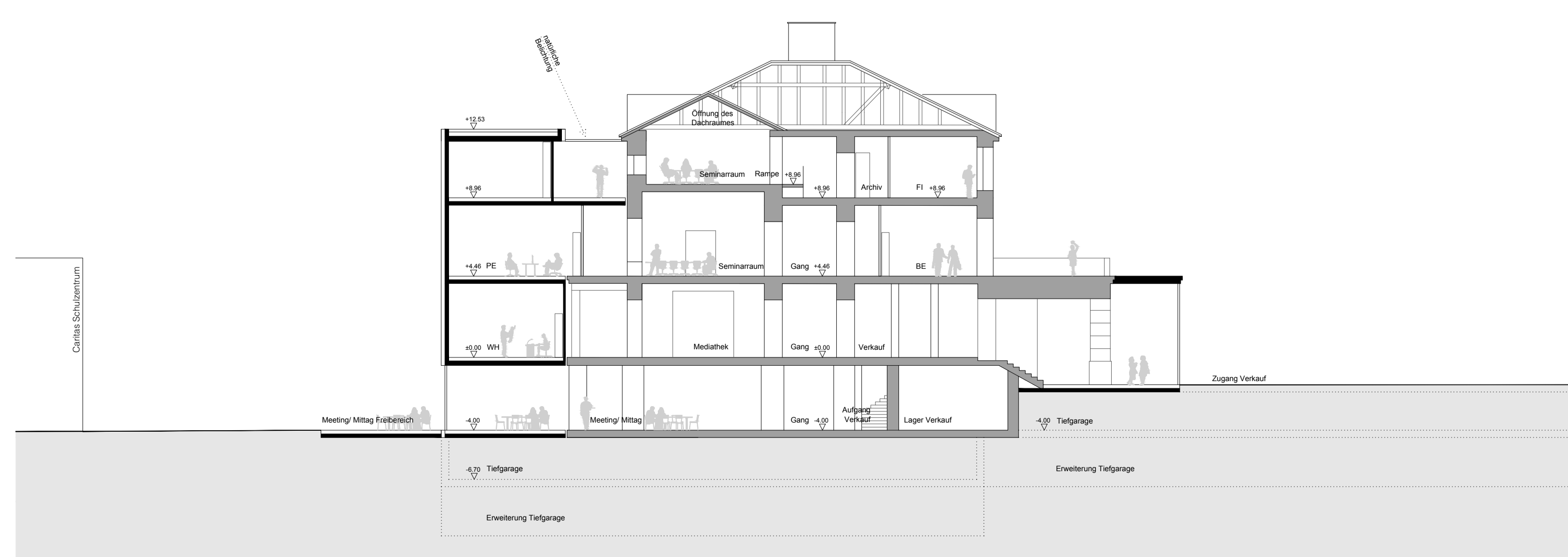
SCHNITT 3-3 1|200
