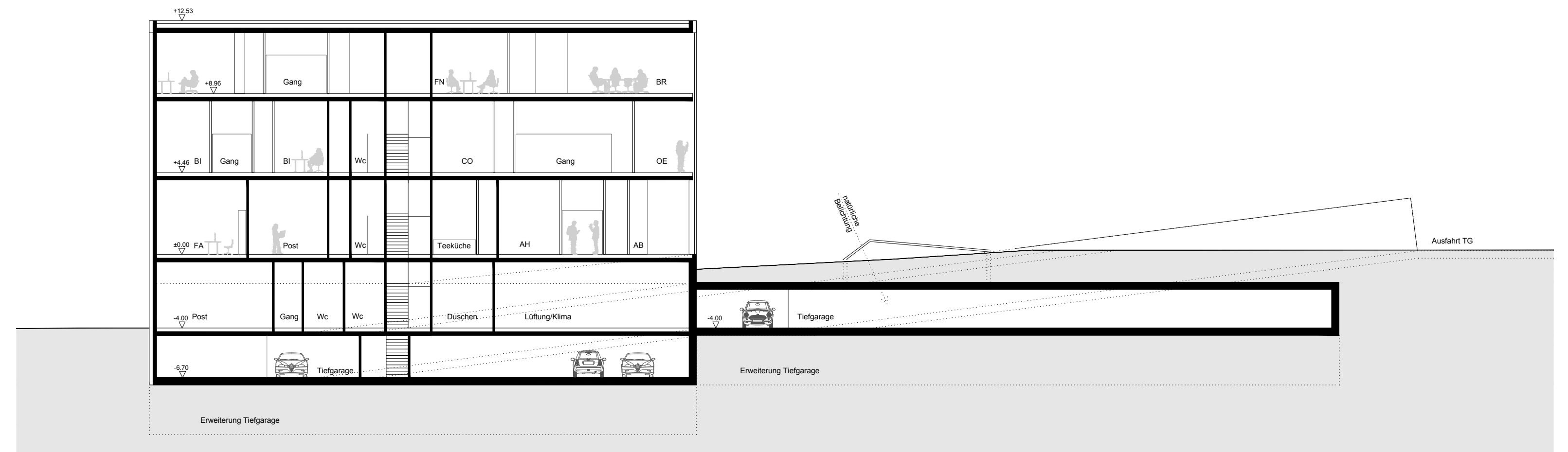
SCHNITT 2-2 1|200
