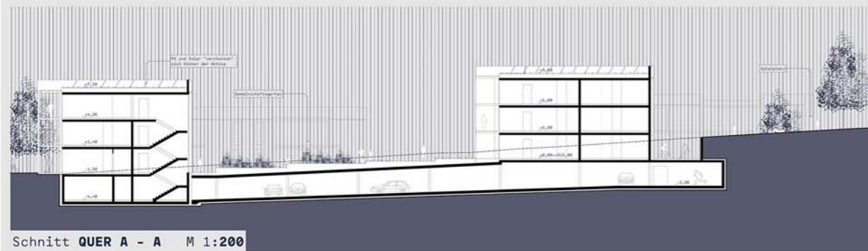
Schnitt QUER A - A M 1:200
