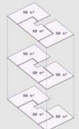
Eigentumswohnungen Haus 02 M 1:100
