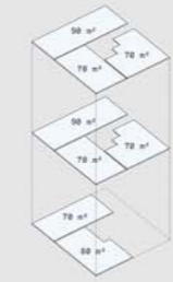
Eigentumswohnungen Haus 01 M 1:100
