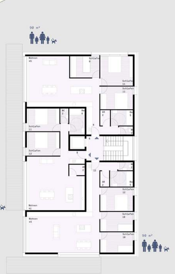
Eigentumswohnungen Haus 02 M 1:100
