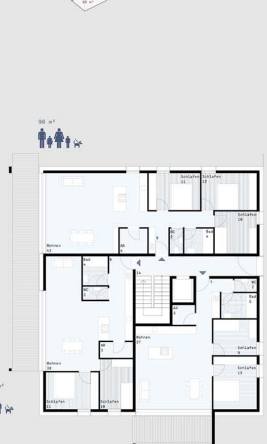
Eigentumswohnungen Haus 01 M 1:100
